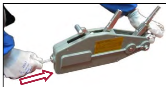
Figura 8 – Inserimento della fune d'acciaio.
