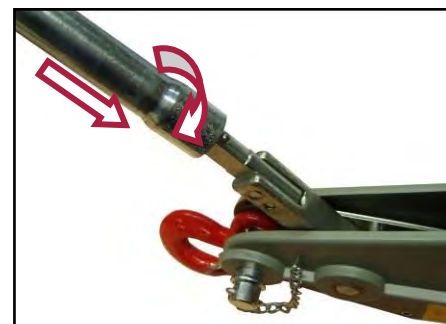
Figura 12 – Inserimento dell'asta sulla leva A.
