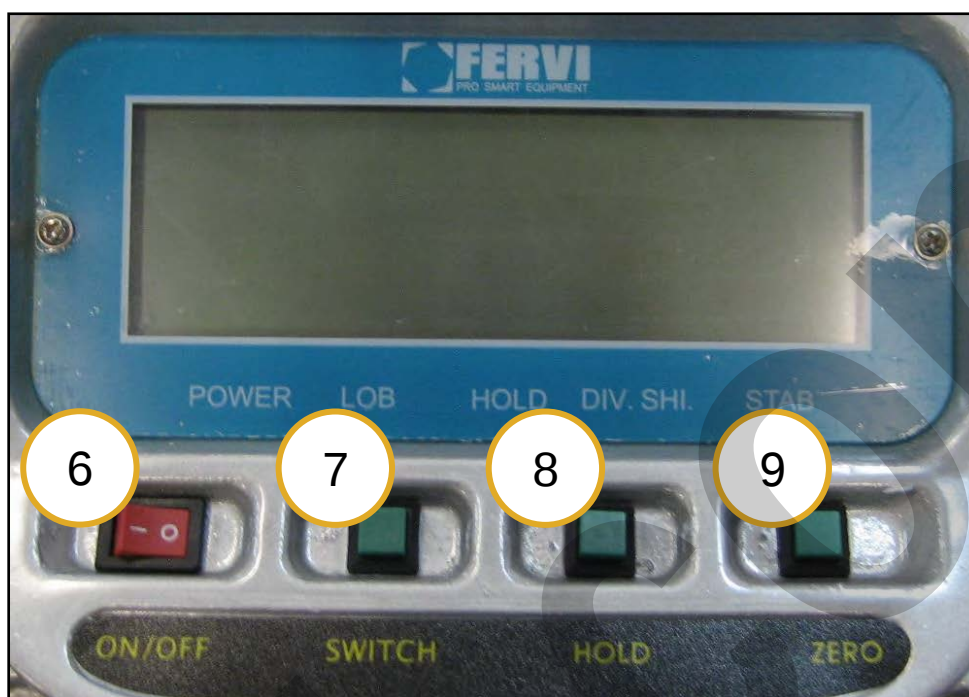
Figura 2 – Dettaglio comandi.
