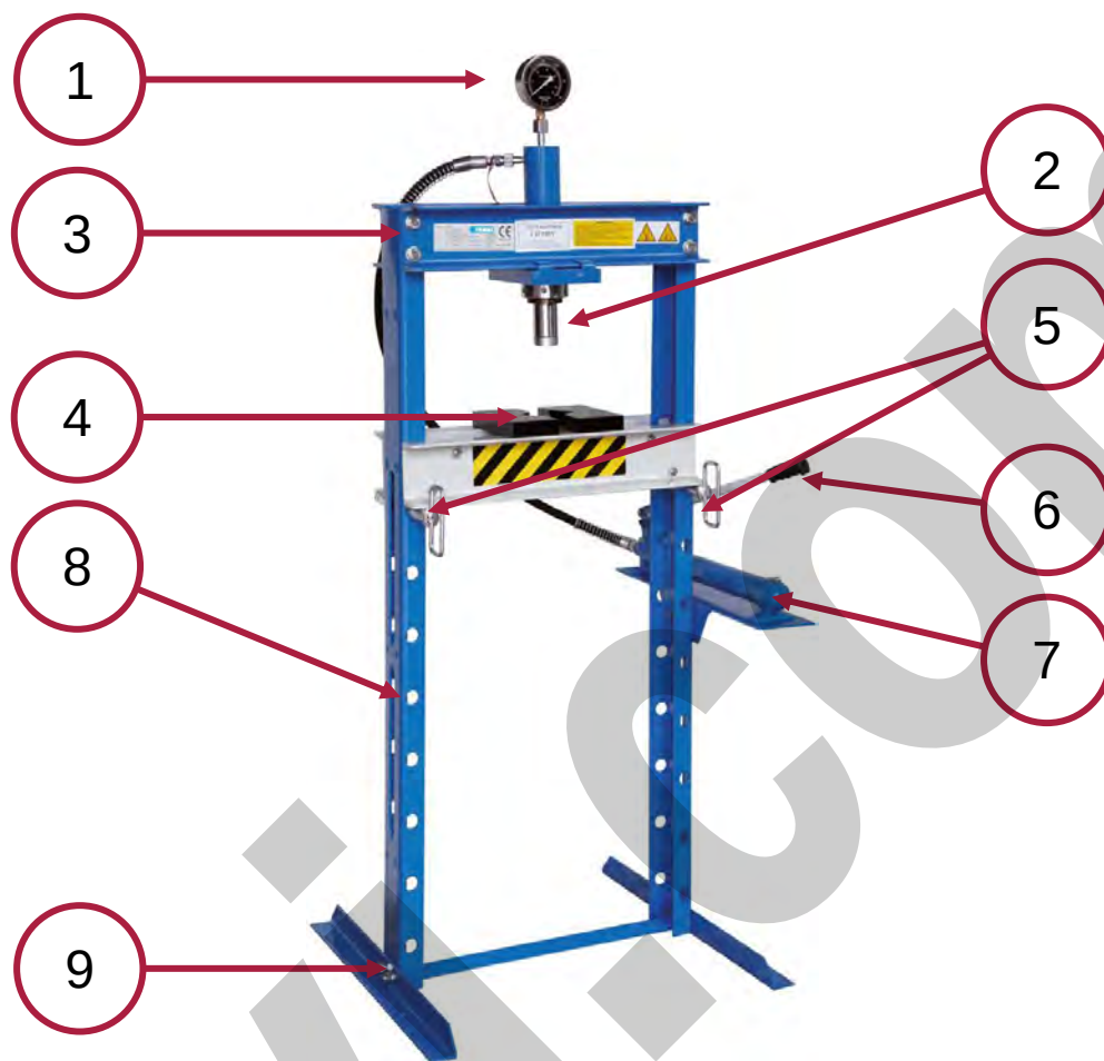
Figura 1 - Parti principali Art. P001/20.
