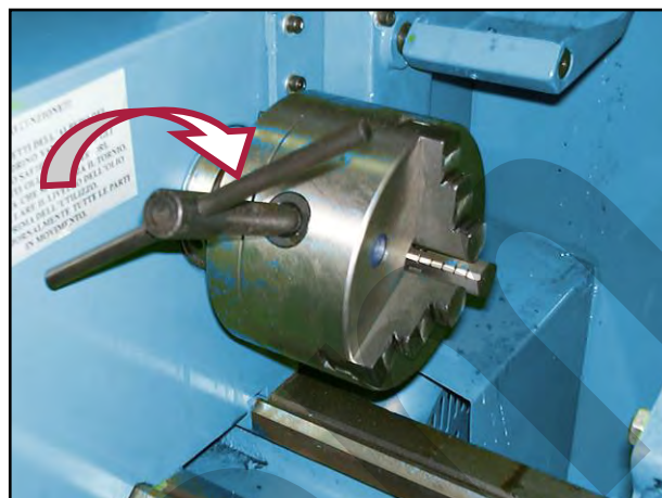
Figura 31 – Chiave del mandrino.
